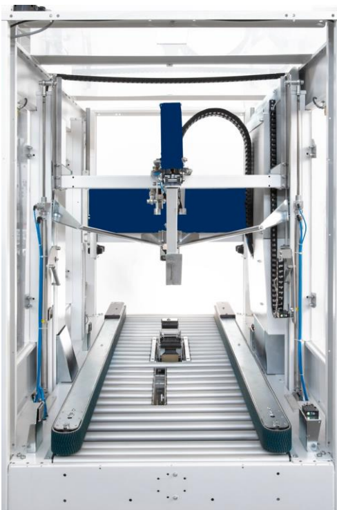
A CT 305 SDRF belső nézete
